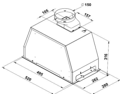
Габаритные размеры вытяжки D 565 S/W/B:
