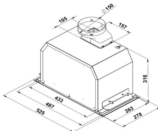
Габаритные размеры вытяжки D 540 S/W/B:
