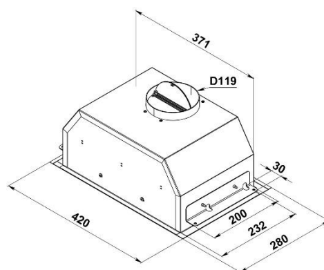
Габаритные размеры вытяжки D 520 S/W/B:
