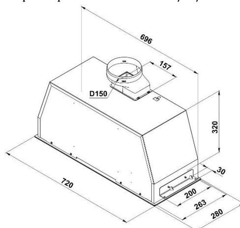
Габаритные размеры вытяжки D 520 S/W/B:
