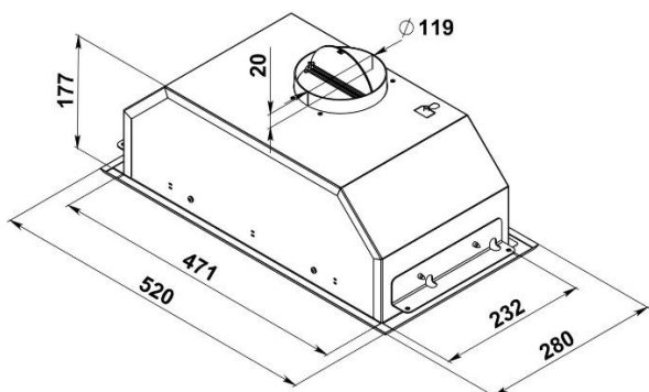
Габаритные размеры вытяжки D 530-549 S/W/B:
