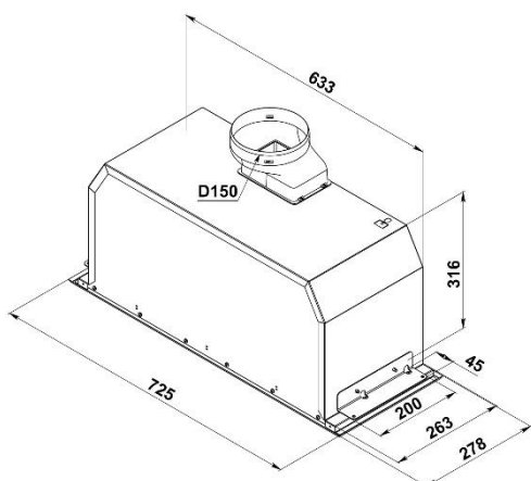
Габаритные размеры вытяжки D 565 S/W/B:
